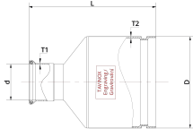
Технічне креслення
