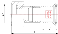
Технічне креслення
