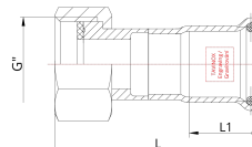
Технічне креслення
