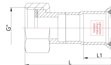
Технічне креслення
