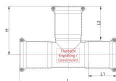
Технічне креслення
