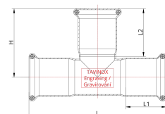
Технічне креслення
