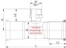
Технічне креслення
