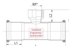
Технічне креслення
