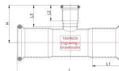
Технічне креслення
