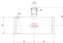
Технічне креслення
