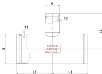
Технічне креслення
